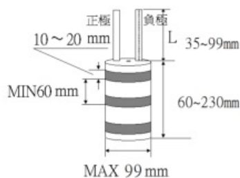
素子尺寸圖
