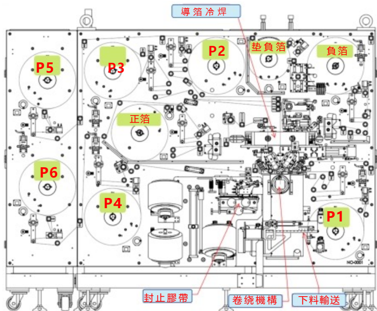
SPHT-1600K-6A配置圖
