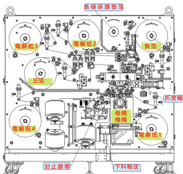
SPHT-1600K-4A配置圖
